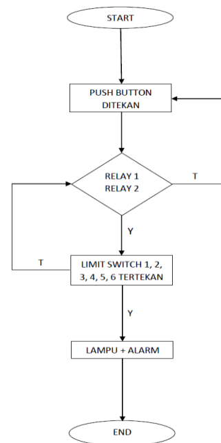
Gambar 9 Flowchart Sistem Keamanan Rumah Menggunakan Relay
