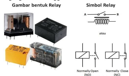
Gambar 1. Bentuk Relay dan Simbol Relay
