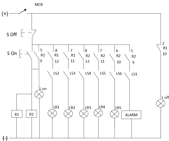
Gambar 8 Rangkaian Kelistrikan Sistem
