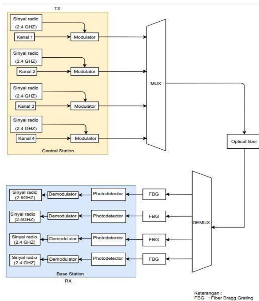
Gambar 2. Konfigurasi Sistem
