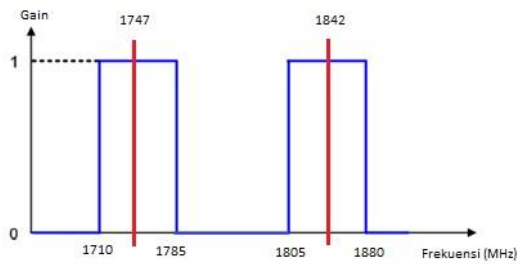
Gambar 3: Respon spesifikasi dualband BPF frekuensi 1800 MHz.
