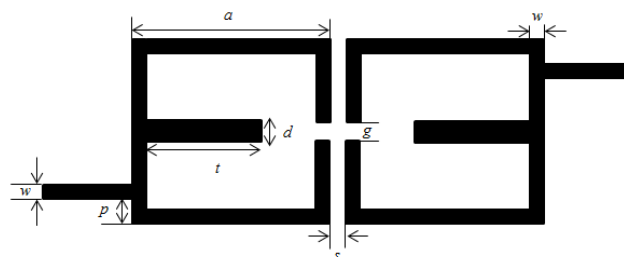
Gambar 5: Desain dualband bandpass filter yang dipergunakan.
