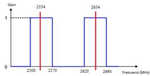
Gambar 4: Respon spesifikasi dualband BPF frekuensi 2600 MHz.
