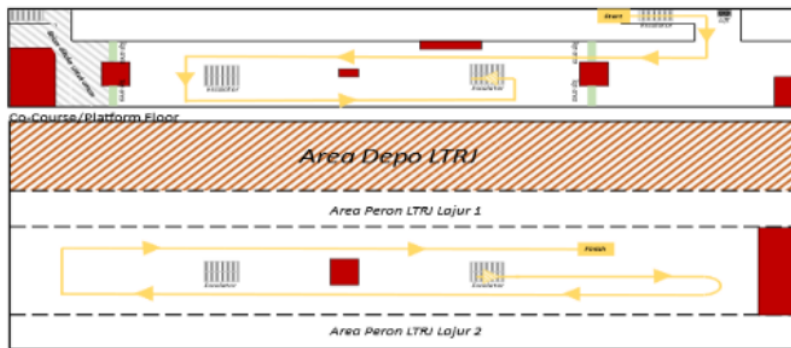
Gambar 5. Rute walk-test Stasiun Pegangsaan Dua
