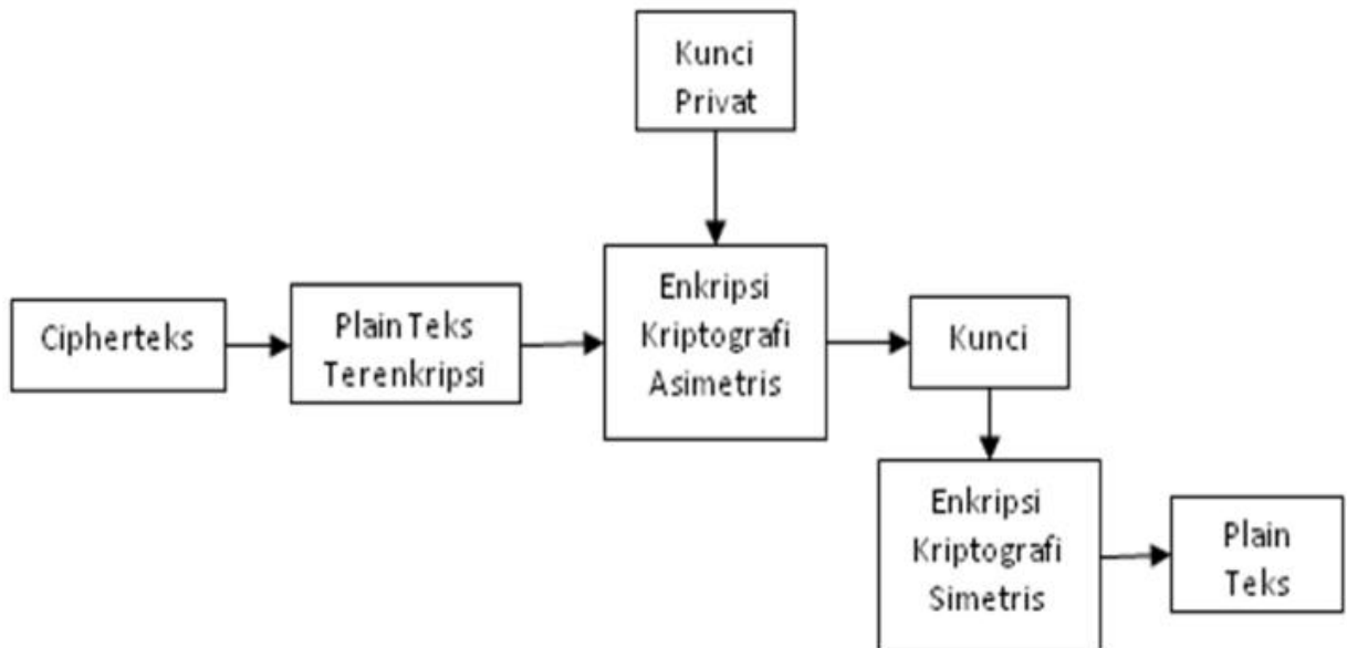
Gambar 5 Dekripsi Dengan Kunci Privat
