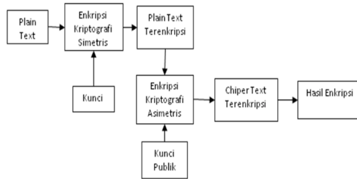
Gambar 4 Enkripsi dengan Kunci Publik
