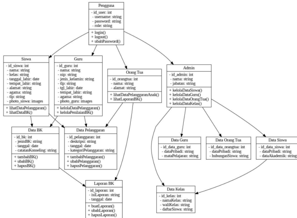
Gambar 3. Perancangan Class Diagram Sistem Informasi Bimbingan Konseling
