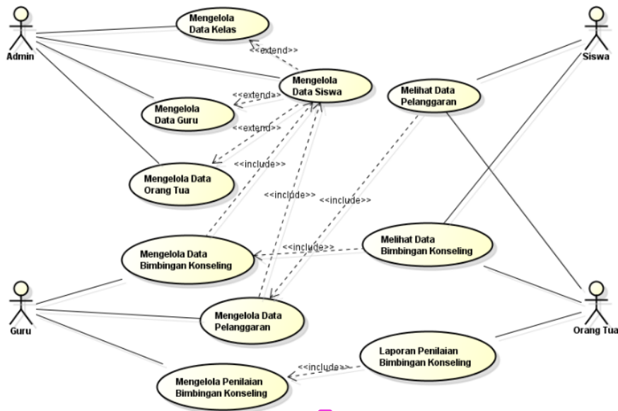
Gambar 2. Perancangan Use Case Diagram Sistem Informasi Bimbingan Konseling
