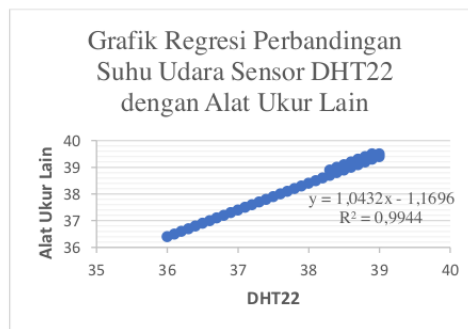
Gambar 6. Kurva Regresi Linear Hasil Pengukuran Suhu
