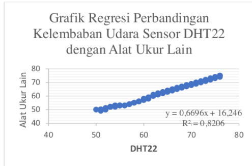
Gambar 8. Kurva Regresi Linear Hasil Pengukuran Kelembaban Udara
