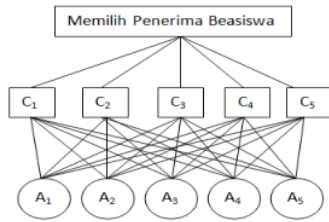
Gambar 1 Struktur Hirarki
