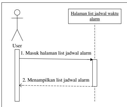
Gambar 8. Sequence Diagram Menampilkan Jadwal Alarm
