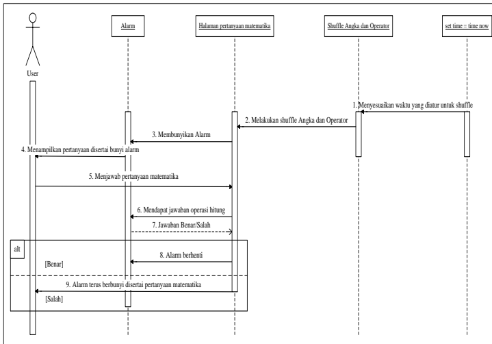
Gambar 10. Sequence Diagram Menjawab Pertanyaan
