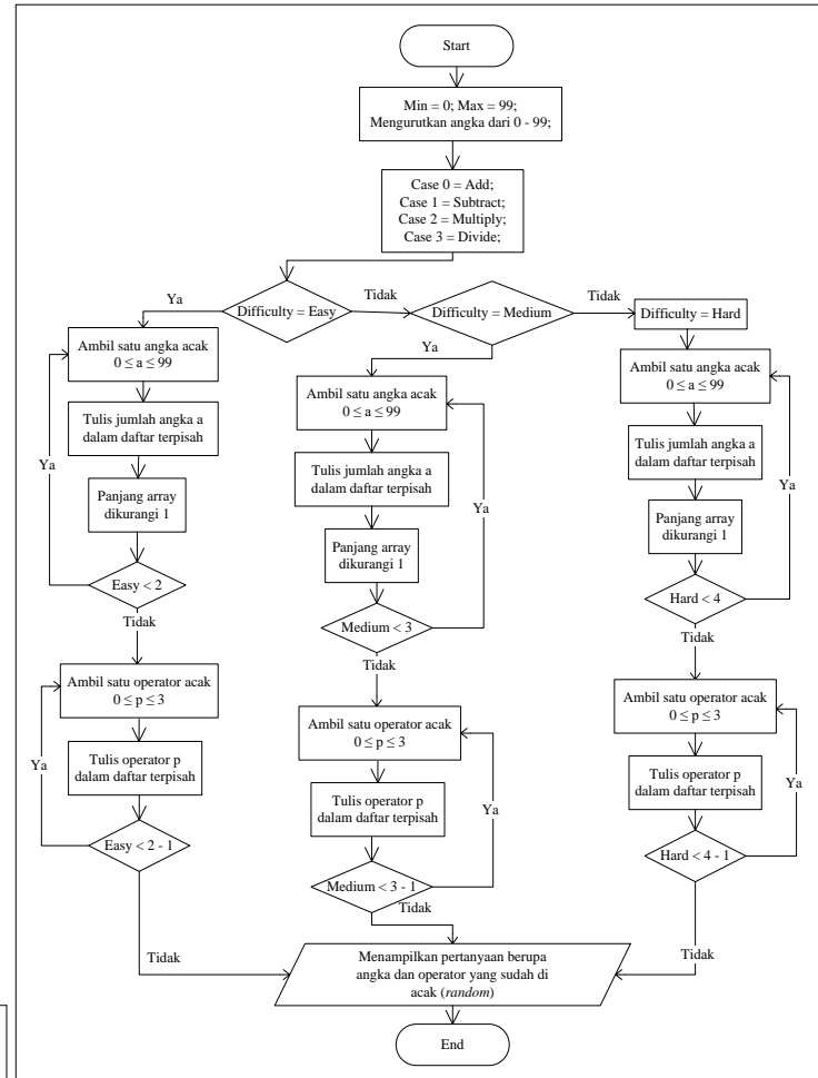
Gambar 12. Flowchart mengacak Angka dan Operator
