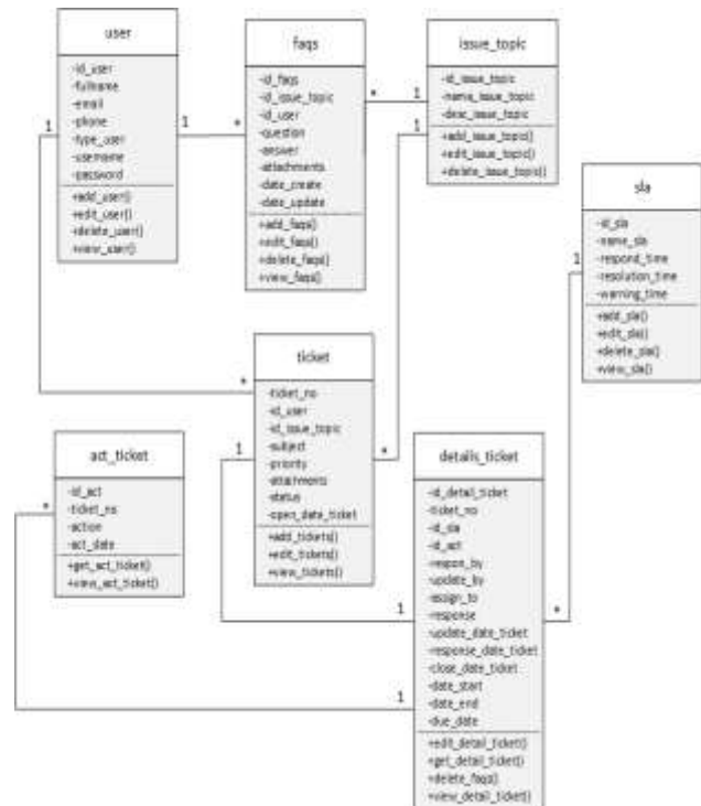
Gambar 7 Class Diagram aplikasi helpdesk ticketing
