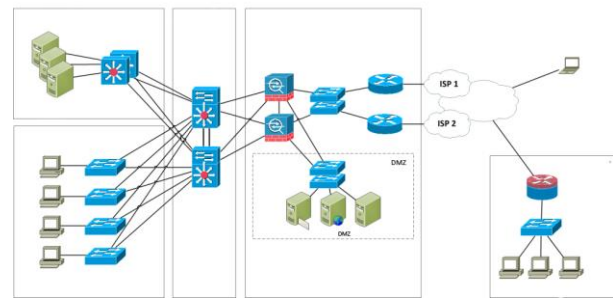
Gambar 3. Topologi Jaringan
