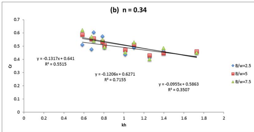
Gambar 9. Hubungan antara koefisien refraksi C_r dengan kedalaman air h , panjang gelombang L , lebar batu pengisi B , lebar balok kotak w dan porositas batu
