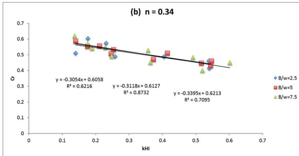
Gambar 8: Hubungan antara koefisien refraksi C_r dengan tinggi gelombang datang H_i , panjang gelombang L , lebar batu pengisi B , lebar balok kotak w dan porositas
