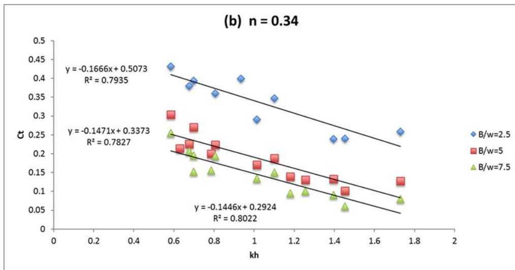
Gambar 7: Hubungan antara koefisien transmisi C_t dengan kedalaman air h , panjang gelombang L , lebar batu pengisi B , lebar balok kotak w dan porositas
