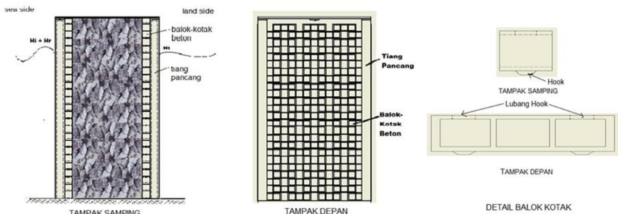
Gambar 1: Sketsa model pemecah gelombang komposit tiang, balok kotak dan batu.
