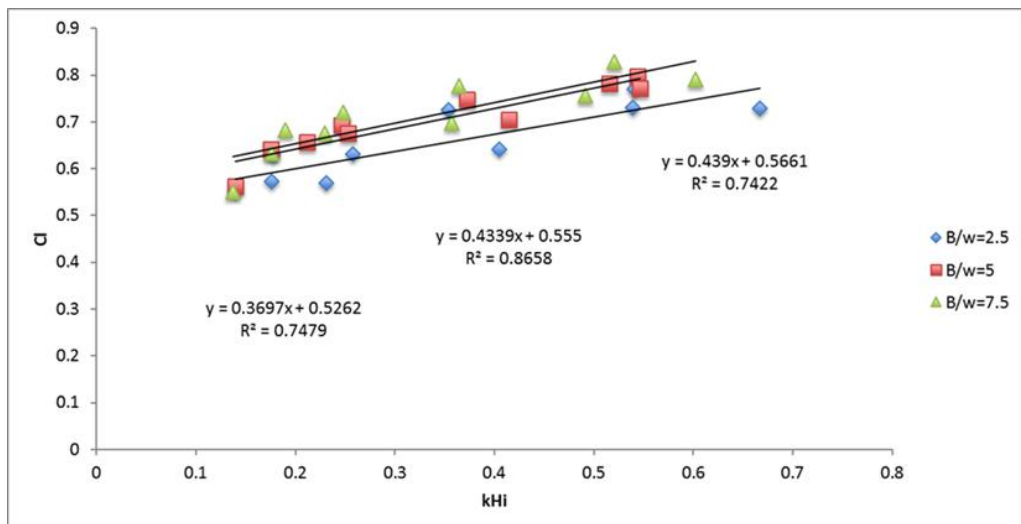
Gambar 10. Hubungan antara koefisien kehilangan energi C_1 dengan tinggi gelombang datang H_i , panjang gelombang L , lebar batu pengisi B , lebar balok kotak w dan porositas batu n konstan.
