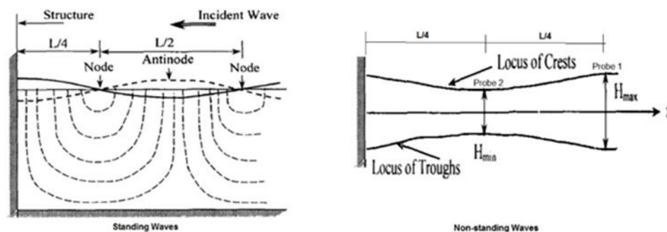
Gambar 3: Posisi Probe 1 dan Probe 2 untuk mengukur H_{max} dan H_{min}
