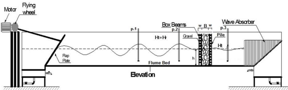
Gambar 2: Sketsa potongan memanjang wave flume yang digunakan dengan posisi model dan instrumentasi.
