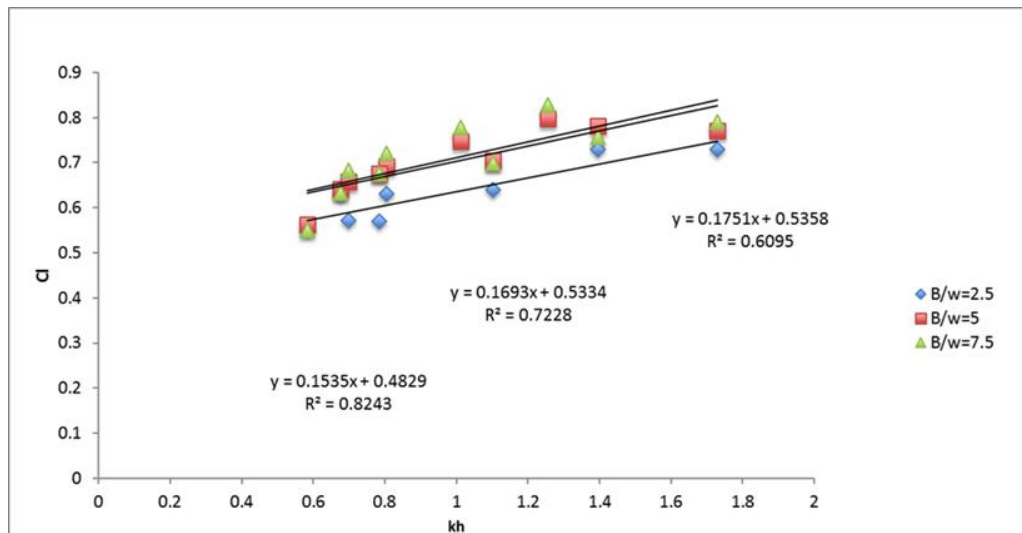
Gambar 11. Hubungan antara koefisien refraksi C_1 dengan kedalaman air h , panjang gelombang L , lebar batu pengisi B , lebar balok kotak w dan porositas batu n konstan.
