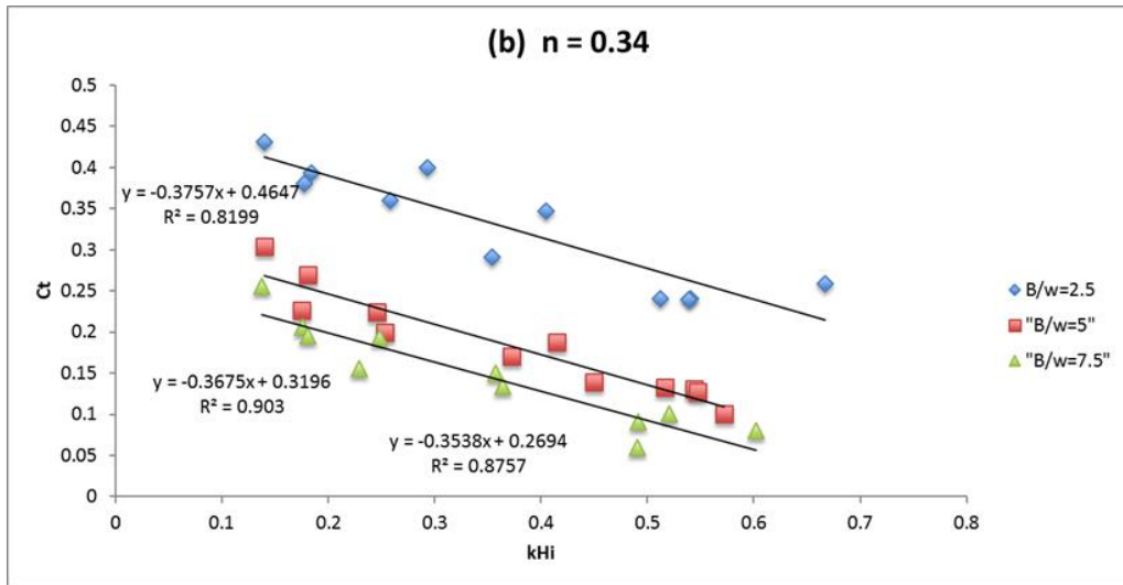
Gambar 6: Hubungan antara koefisien transmisi C_t dengan tinggi gelombang datang H_i , panjang gelombang L , lebar batu pengisi B , lebar balok kotak w dan porositas batu n .
