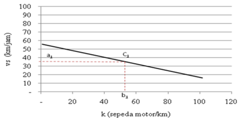
Gambar 17. Penentuan nilai kapasitas ( C_1 ) arah Surabaya
