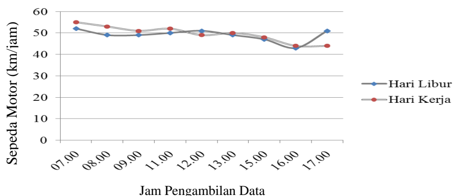
Gambar 9. Grafik data kecepatan tempuh di JKSM arah Madura
