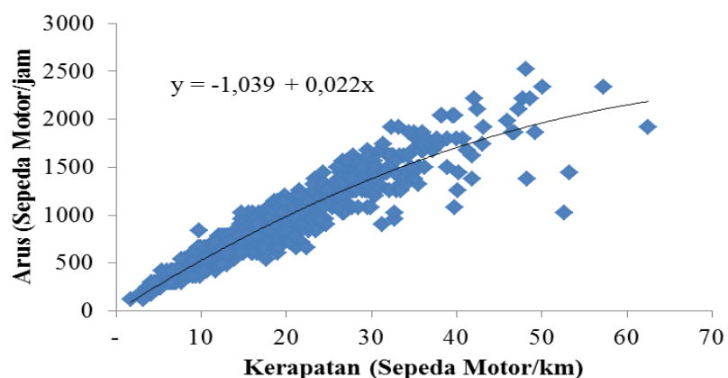
Gambar 13. Hubungan antara kerapatan dan arus di JKSM Jalan Tol Suramadu Arah Madura
