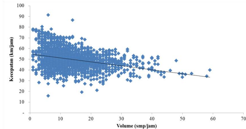
Gambar 10. Hubungan volume sepeda motor dan kecepatan tempuh
