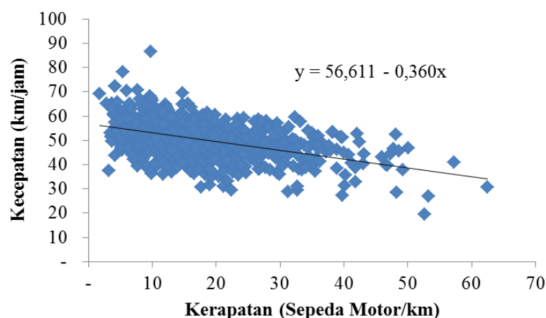
Gambar 11. Hubungan Antara Kerapatan dan Kecepatan tempuh di JKSM Jalan Tol Suramadu Arah Madura
