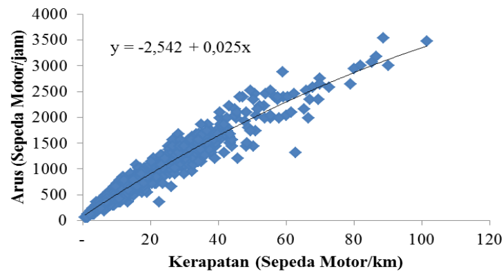
Gambar 14. Hubungan antara kerapatan dan arus di JKSM Jalan Tol Suramadu arah Surabaya
