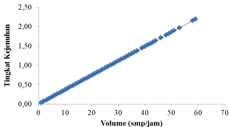
Gambar 19. Hubungan antara volume sepeda motor dengan tingkat kejenuhan
