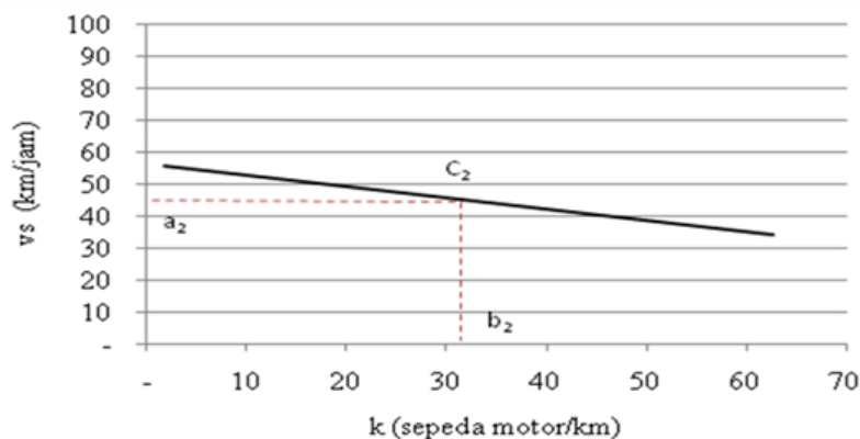
Gambar 18. Penentuan nilai kapasitas ( C_2 ) arah madura
