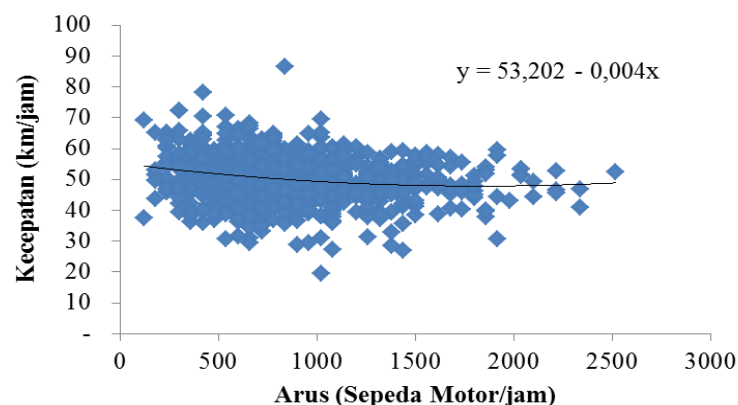
Gambar 15. Hubungan antara kecepatan tempuh dan arus di JKSM Jalan Tol Suramadu arah Madura
