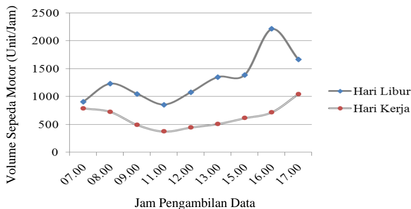
Gambar 6. Grafik data volume di JKSM arah Surabaya
