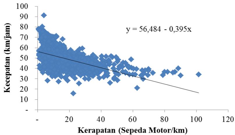
Gambar 12 Hubungan antara kerapatan dan kecepatan tempuh di JKSM Jalan Tol Suramadu arah Surabaya
