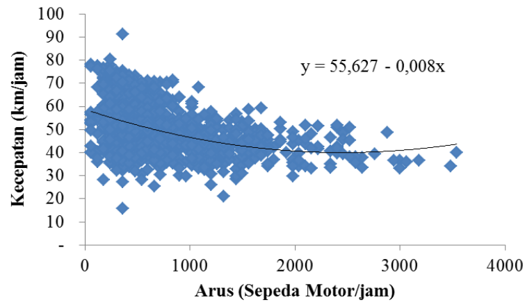
Gambar 16 Hubungan antara kecepatan tempuh dan arus di JKSM Jalan Tol Suramadu arah Surabaya
