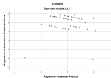
Gambar 1 uji heteroskedastisitas variabel penghambat
