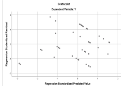
Gambar 2 uji heteroskedastisitas variabel pendorong
