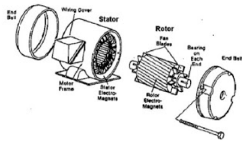
Gambar 4 Motor Induksi
