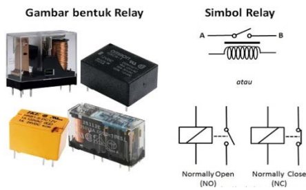
Gambar 2. Gambar Bentuk dan Simbol Relay
