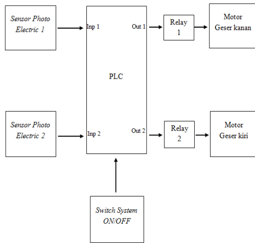
Gambar 6 Diagram Perancangan Kendali
