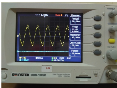
Gambar 4.6 Hasil pengukuran sinyal yang di terima oleh photodiode
