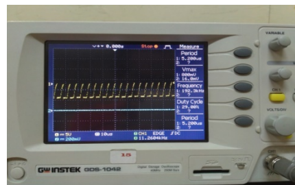
Gambar 4.3 Hasil pengukuran VCO menggunakan osiloscope
