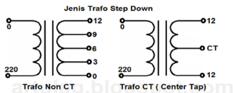
Gambar 2.7 Trafo step down
