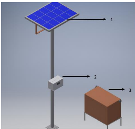
Gambar 2. Desain Prototype Pelindung Rumput Laut
