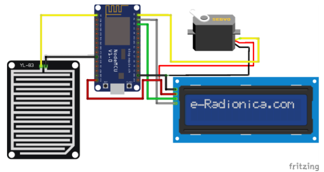
Gambar 3. Rangkaian Keseluruhan
