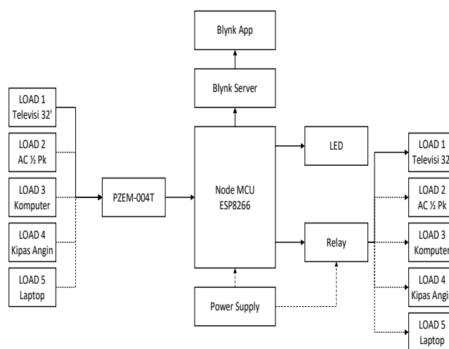
Gambar 1. Blok Diagram Rangkaian
