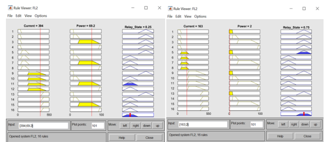
Gambar 16. Simulasi Matlab Fuzzy Logic Beban Komputer
