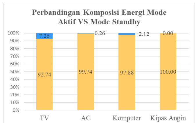
Gambar 19. Perbandingan komposisi energi mode aktif dan standby
