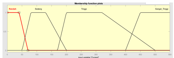
Gambar 6. Kurva Himpunan Fuzzy Input Arus
