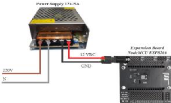
Gambar 2. Rangkaian Catudaya
