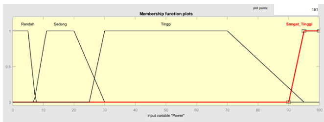
Gambar 7. Kurva Himpunan Fuzzy Input Daya Listrik
