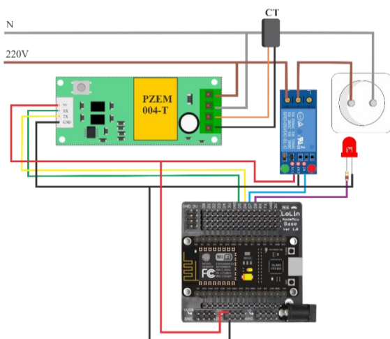
Gambar 3 Rangkaian Sistem
