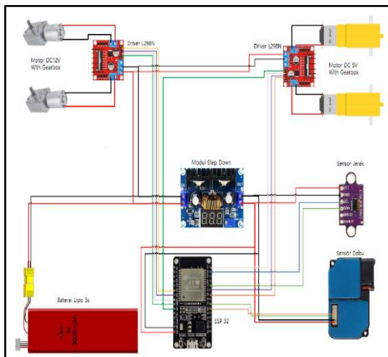
Gambar 4. Rangkaian Skematik
