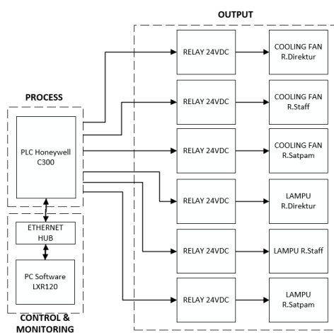
Gambar 1. Diagram Blok Perancangan
