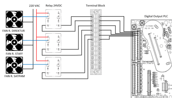
Gambar 4. Diagram Pengawatan Sistem Pendingin
