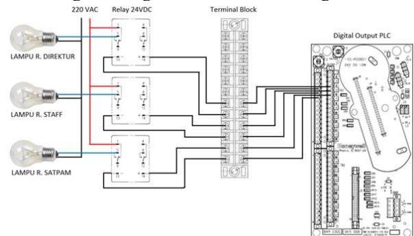
Gambar 5. Diagram Pengawatan Sistem Penerangan
