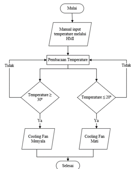
Gambar 2. Diagram Alir Sistem Pendinginan
