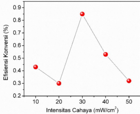
Gambar 2. Efisiensi konversi fotovoltaik terhadap intensitas cahaya
