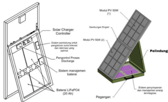
Gambar 1. Skematik sistem Integrasi fotovoltaik dalam bentuk portabel
