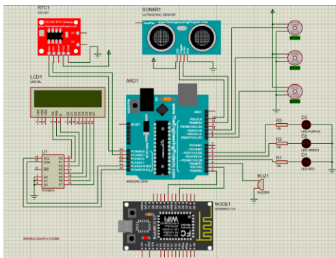
Gambar 3. Perancangan Elektronik
