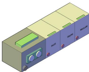
Gambar 4. Perancangan Mekanik
