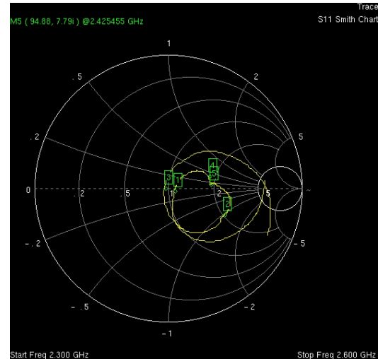
Gambar 8 : Pengukuran Impedansi Masukan Dengan Network Analyzer
