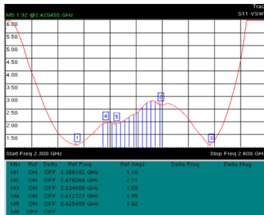
Gambar 7 : Pengukuran VSWR Dengan Network Analyzer
