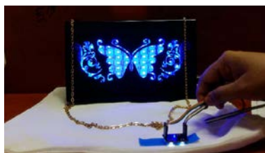
Gambar 4.11 Pengujian sensor warna terhadap kertas warna biru
