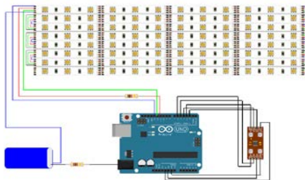
Gambar 4.3 Rangkaian Sensor Warna
