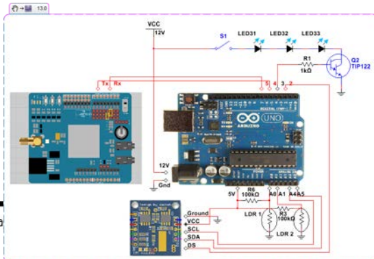
Gambar 2. Rangkaian Lengkap
