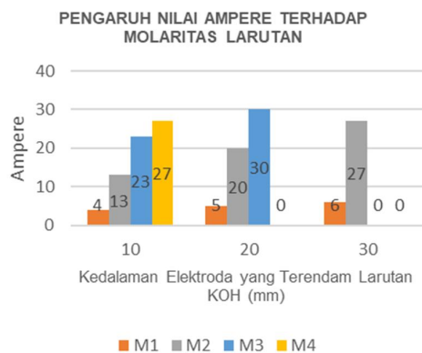
Gambar 6. Diagram pengaruh nilai ampere terhadap molaritas larutan
