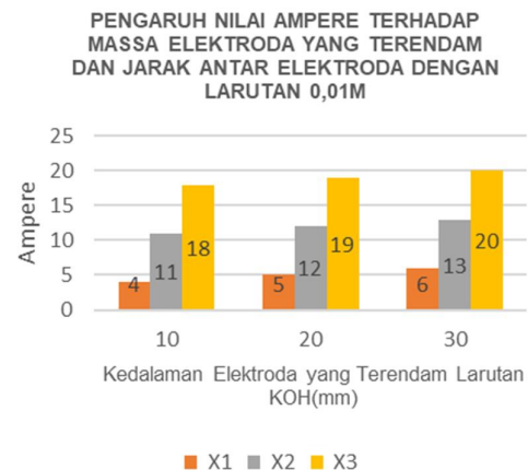
Gambar 5. Diagram pengaruh nilai ampere terhadap massa elektroda yang terendam dan jarak antar elektroda
