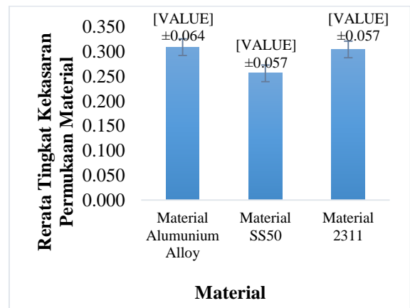
Gambar 6. Grafik Rata-rata Tingkat Kekasaran Permukaan Material
