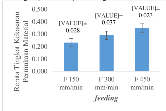
Gambar 7. Grafik Rata-rata Tingkat Kekasaran Permukaan Material
