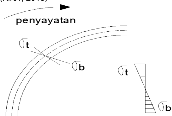
Gambar 1. Ilustrasi Tegangan pada Penampang Total
