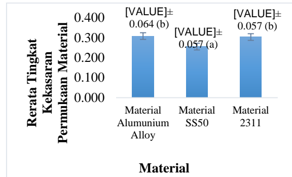
Gambar 8. Grafik Rerata Tingkat Kekasaran Permukaan Material
