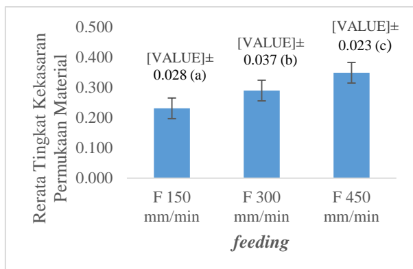
Gambar 9. Grafik Rata-rata Tingkat Kekasaran Permukaan Material
