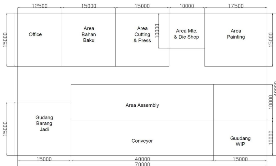
Gambar 12 Layout Usulan.
