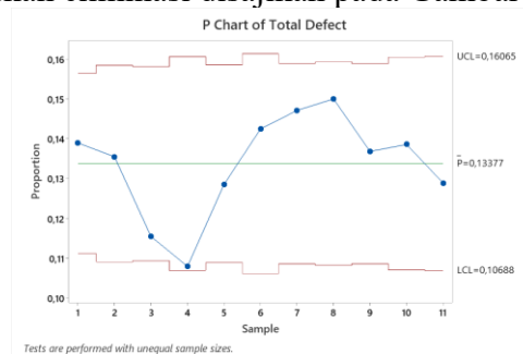
Gambar 4. Peta Kendali P Produk Valve Perbaikan
