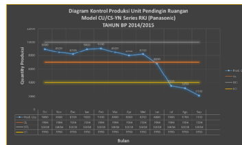
Gambar 3. Diagram Kontrol Produksi Tahun BP 2015 / 2016
