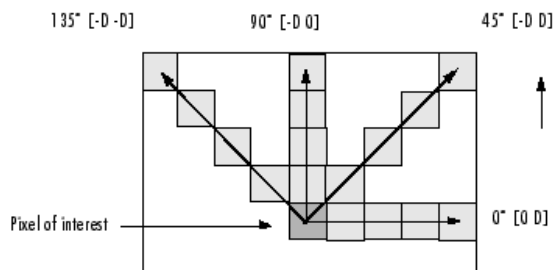
Gambar 1. Empat Arah Derajat Keabuan
