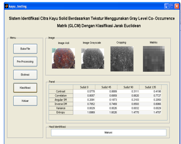
Gambar 6. GUI Sistem Identifikasi Kayu Solid
