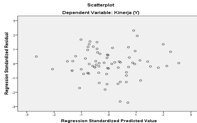
Gambar 1. Uji Heteroskedastisitas
