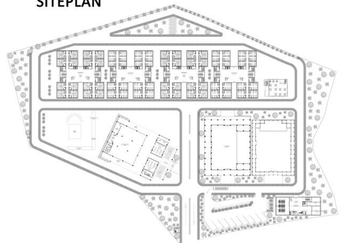
SITEPLAN
