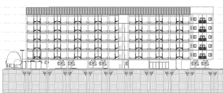
POTONGAN D-D BANGUNAN B 1:200
