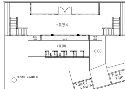
Gambar 2. Siteplan Masjid Al-Karim dan Denah Ruang Wudhu Masjid Al-Karim Sumber : Kurniawan, 2017
